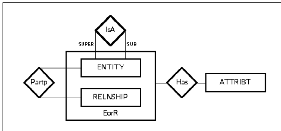
Figure 3. ER Meta-Model for ER Models
